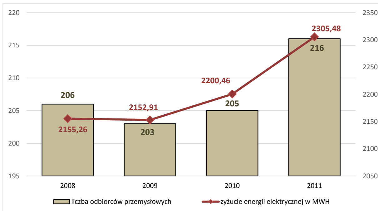
Wykres 3. Zużycie prądu przez odbiorców przemysłowych w latach 2008 - 2011
